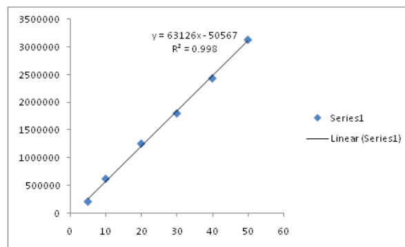
Fig. 5: Linearity graph for EZT
